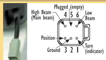
Grommet + 6 pin Deutsch harness
